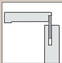
Typ P Designkante R=1,5 mm Bekleidungsbreite 70 mm
